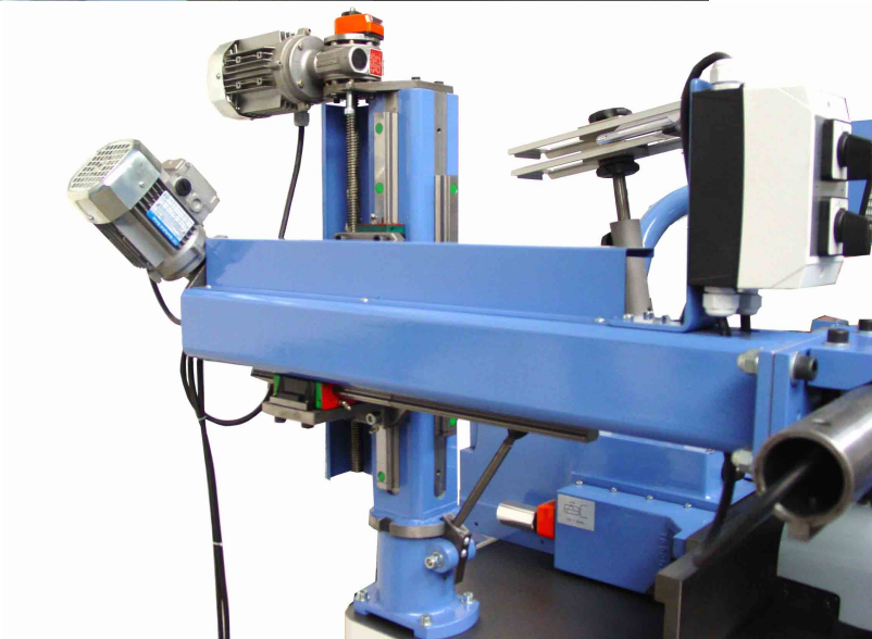
Colonne axe horizontal avec guidages linéaires, moto-reducteur, et système de mesure et indication digitale
